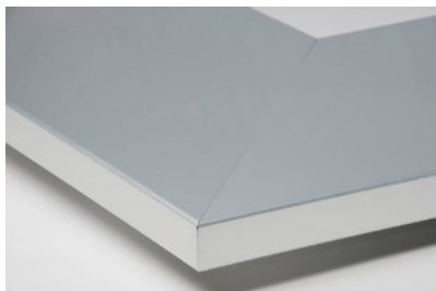
Detail Gehrung 90°
